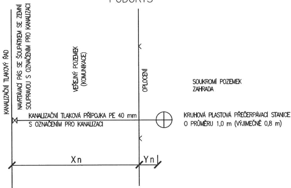
PŮDORYS
