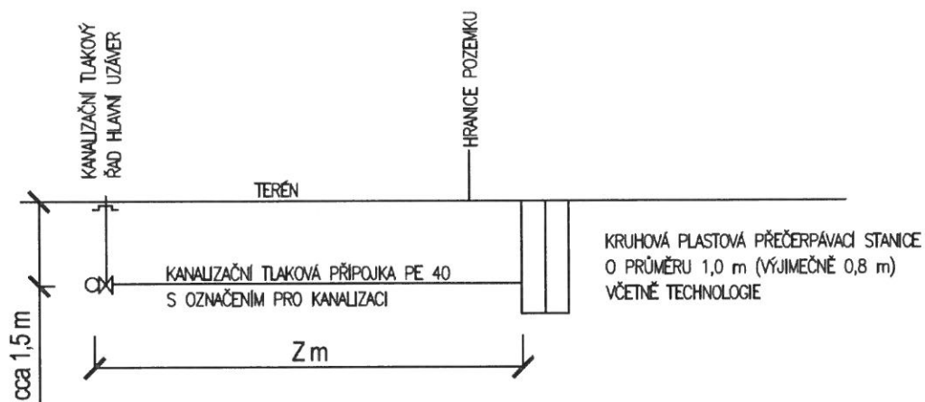
PODÉLNÉ SCHEMA
