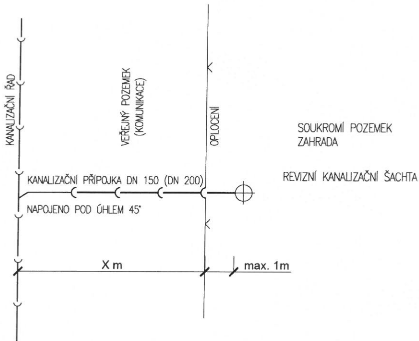
PODÉLNÉ SCHEMA
