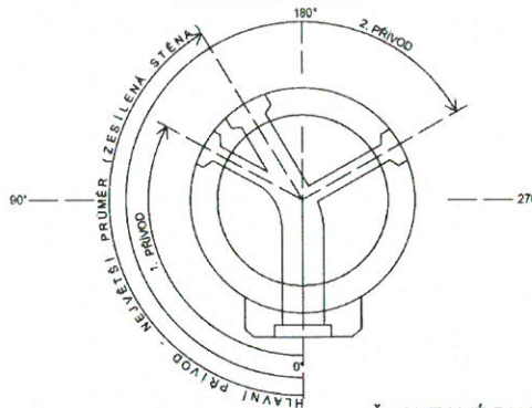
ŠACHTOVÉ DNO S HRDLEM DIN 4034.1 - TZZ-Q 1000/1150
