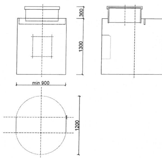
VODOMĚRNÁ ŠACHTA OVÁLNÁ DN 1250
