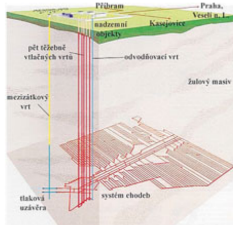
Schéma PZP Háje
