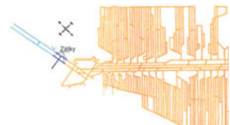
Systém chodeb a tlakové uzávěry
